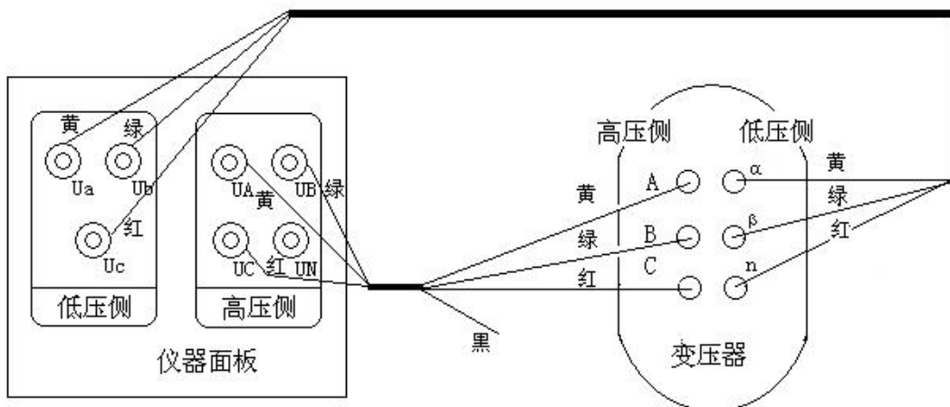
图 21 斯科特型变的测试接线
