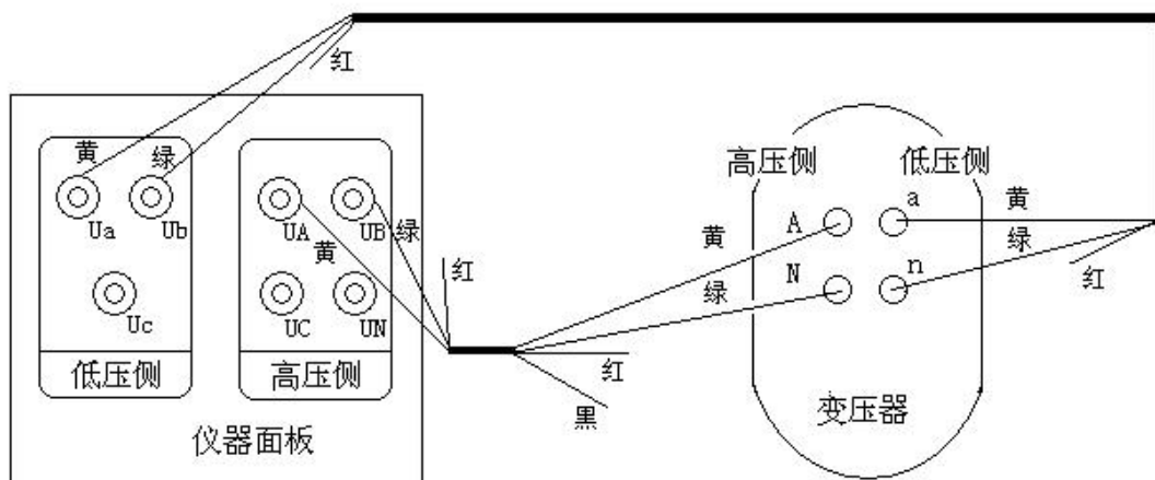
图 20 单相变压器的测试接线
