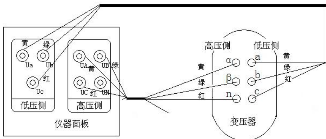
图 21 逆斯科特变压器的测试接线
