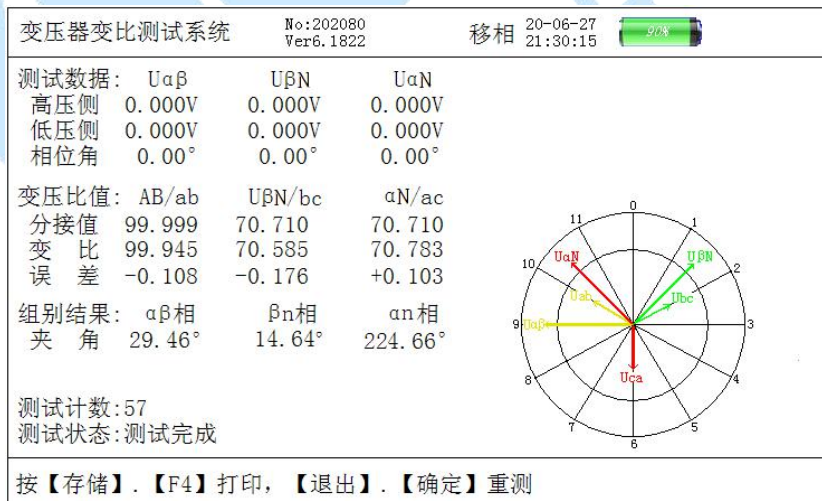
图 17 斯科特变压器测试结果屏
