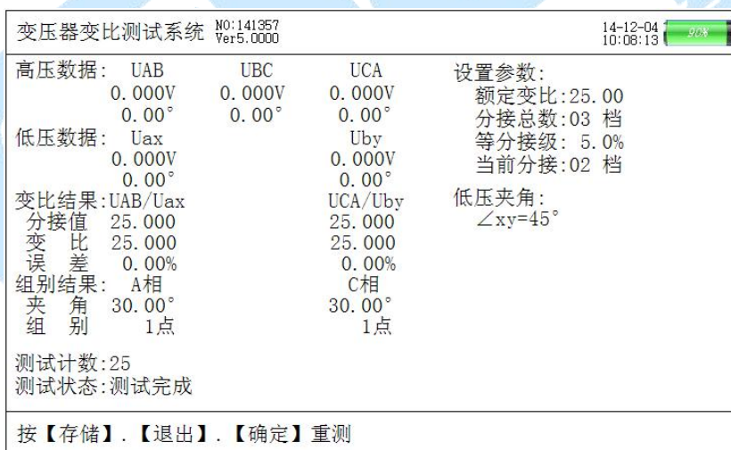
图 15 斯科特变压器测试结果屏
