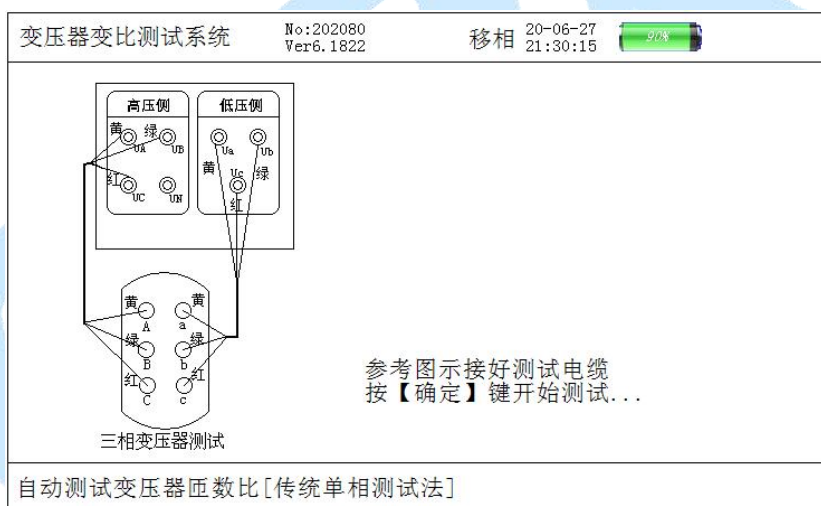
图 8 三相匝数比测试接线提示屏
