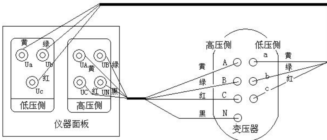
图 21 Z 型变的测试接线
