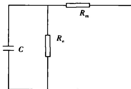
图 1 蓄电池简化等效模型
